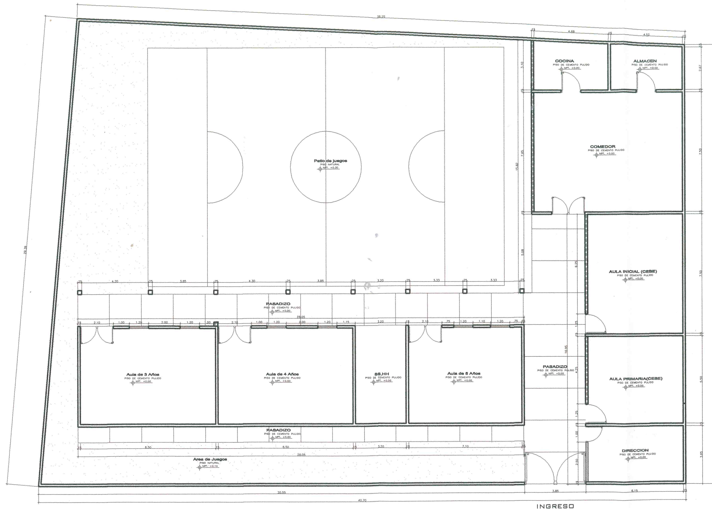
PLANO DE DISTRIBUCION ESC. 1/250
